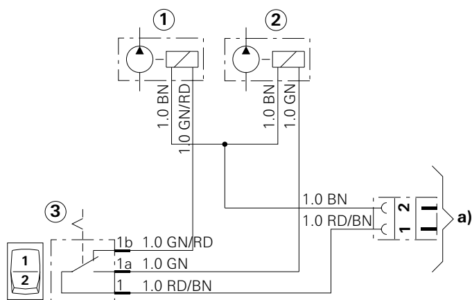
Apertura incorporata per il commutatore senza apertura
