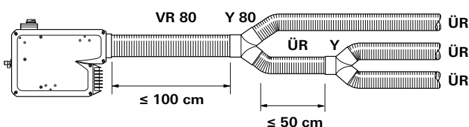
Fig. 18 – eksempel på et varmluftsystem Truma VarioHeat comfort
