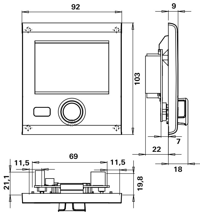
Afbeelding 21 – Afmetingen in mm. Weergave niet op schaal
