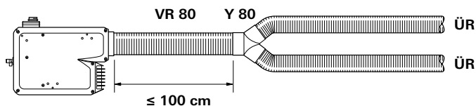
Bild 17 – Exempel varmluftssystem Truma VarioHeat eco
