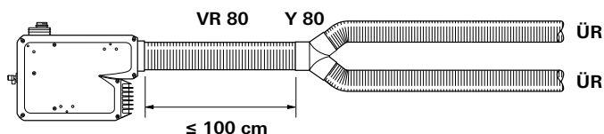
Afbeelding 17 – Voorbeeld warmeluchtsysteem Truma VarioHeat eco
