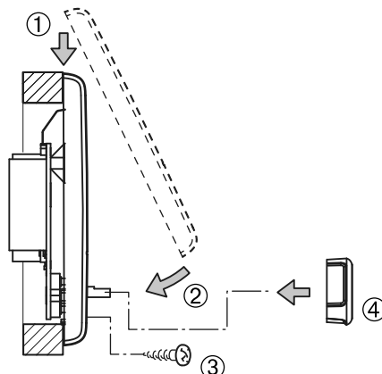
Afbeelding 25 – Kapje bedieningspaneel en draai-/drukknop monteren
