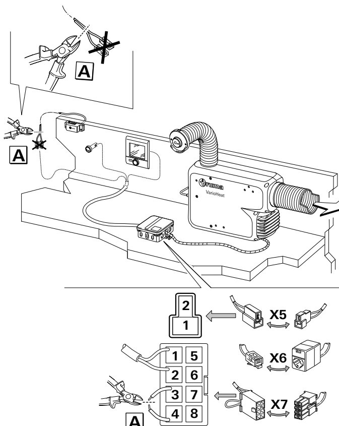
Fig. 27 – tilslutningsdiagram
