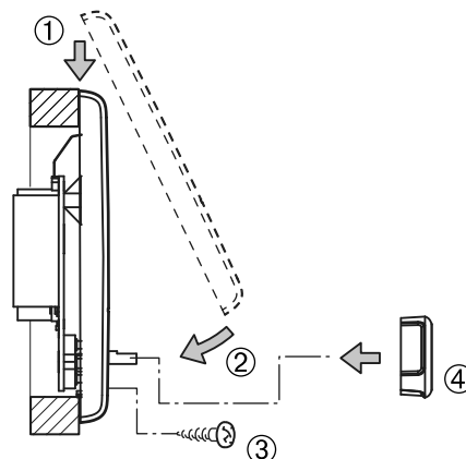
Bild 25 – Montera manöverenhetens överdel och vrid- / tryckknappen
