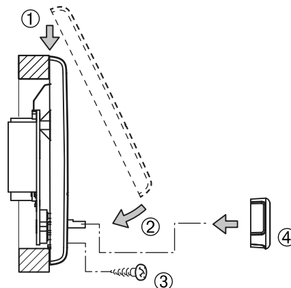
Fig. 25 – Monter betjeningsdelens øverste del og dreje-/trykknappen
