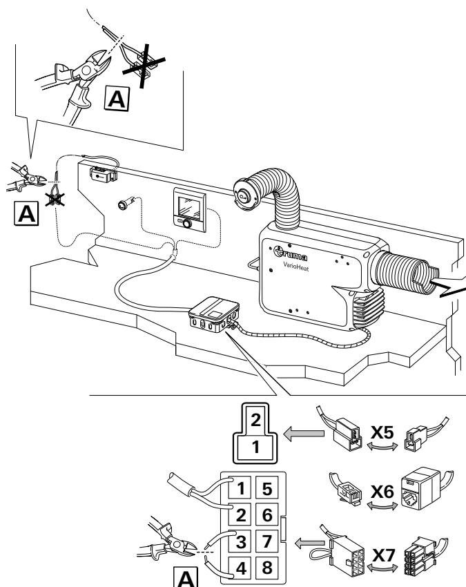
Bild 27 –Kopplingsschema
