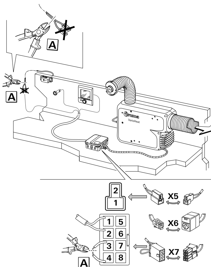
Fig. 27 – schema di collegamento
