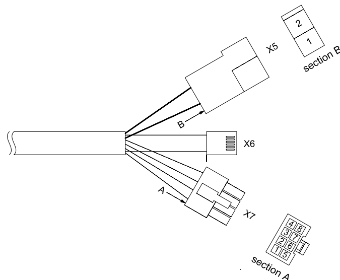
Bild 28 –Kabelstam
