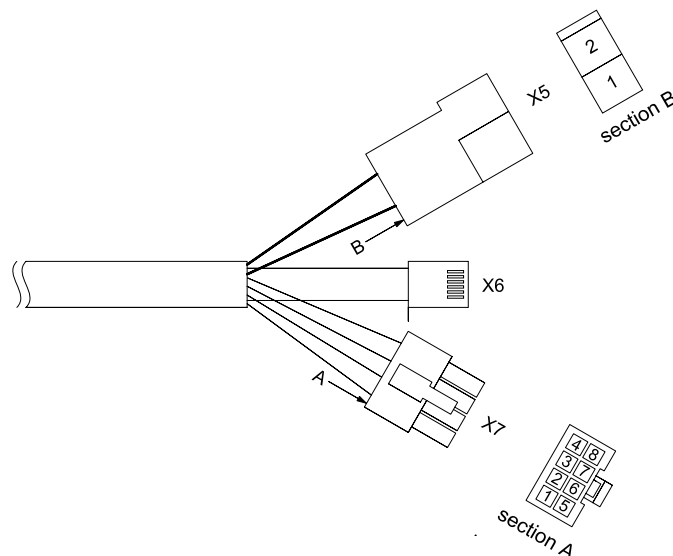
Fig. 28 – cablaggio
