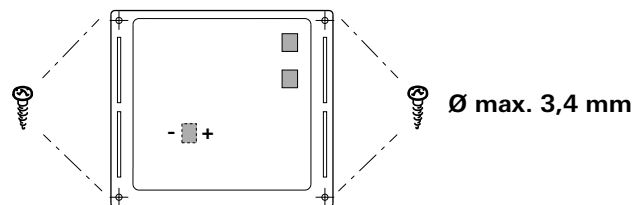
Fig. 24 – set forfra
