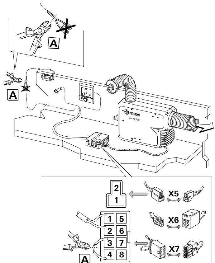
Afbeelding 27 – Aansluitschema
