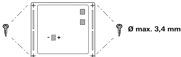
Bild 24 – Vy framifrån
