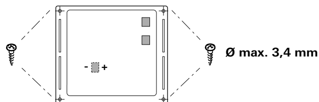
Figura 24 – Vista frontale
