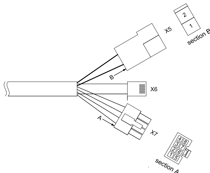
Fig. 28 – kabelbundt
